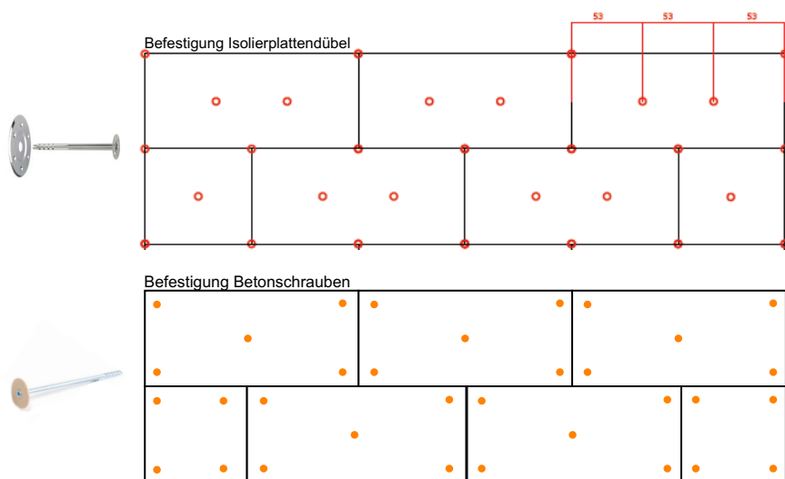
Dübelschema zur nachträglichen Befestigung
