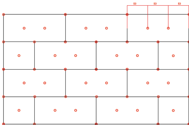
Dübelschema zur nachträglichen Befestigung
